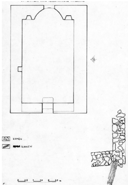
Сл. 4. Темељи цркве из 15. века у односу на савремену цркву (Ерцеговић-Павловић, Костић 1988, 39)
